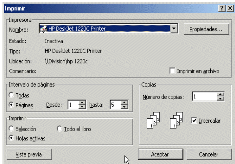
Figura 61. Comando Imprimir .
